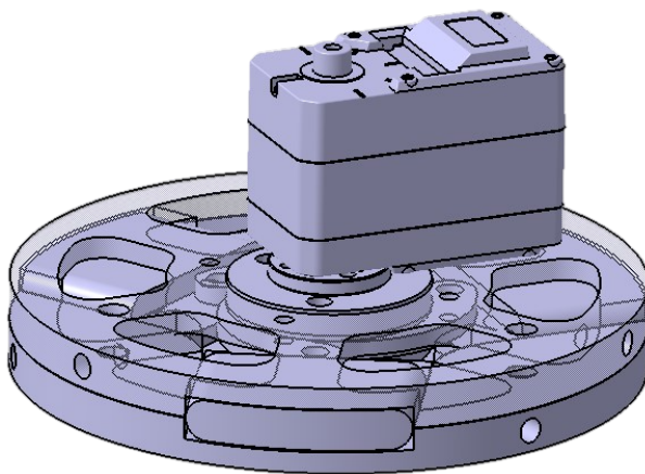
FIGURE 4.3 – Système d'aérofrein d'SP-02 sur CA-TIA
