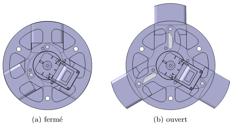
FIGURE 4.4 – Position des aérofreins d'SP-02
